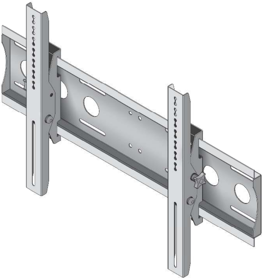
LWB2/PWB2/TWB2 Tilting Wall Mount / Uchylny uchwyt ścienny
