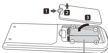
R03/LR03, AAA (Alkali- oder Manganbatterien)
