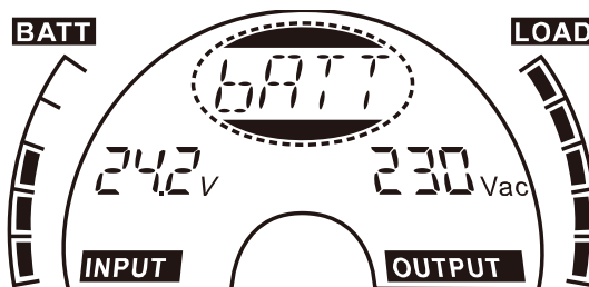
■ Abbildung 6.2 Batteriebetrieb
