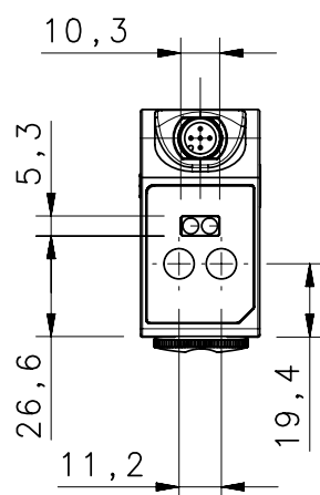
TL46-W/TL46-WJ
