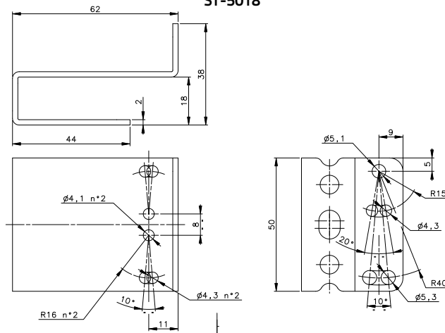
ST-5018
