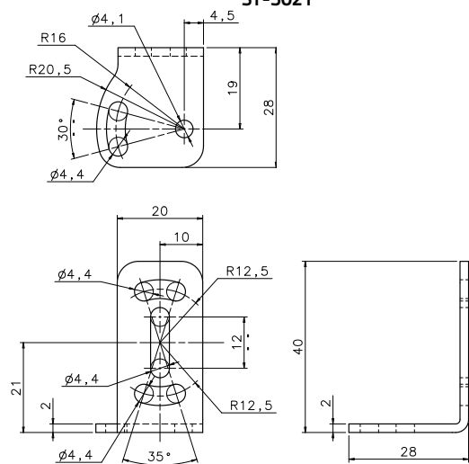
ST-5021
