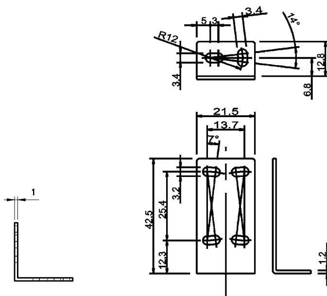
ST-5039
